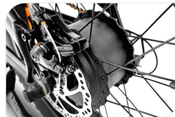
Motore Sutto Bafang 55Nm
