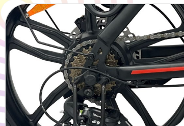
Moteur Sutto Bafang, 250 W, 48 V, 70 Nm
