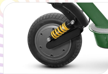
Moteur Brushless, 15 Nm, KERS, Puissance maximale 900 W
